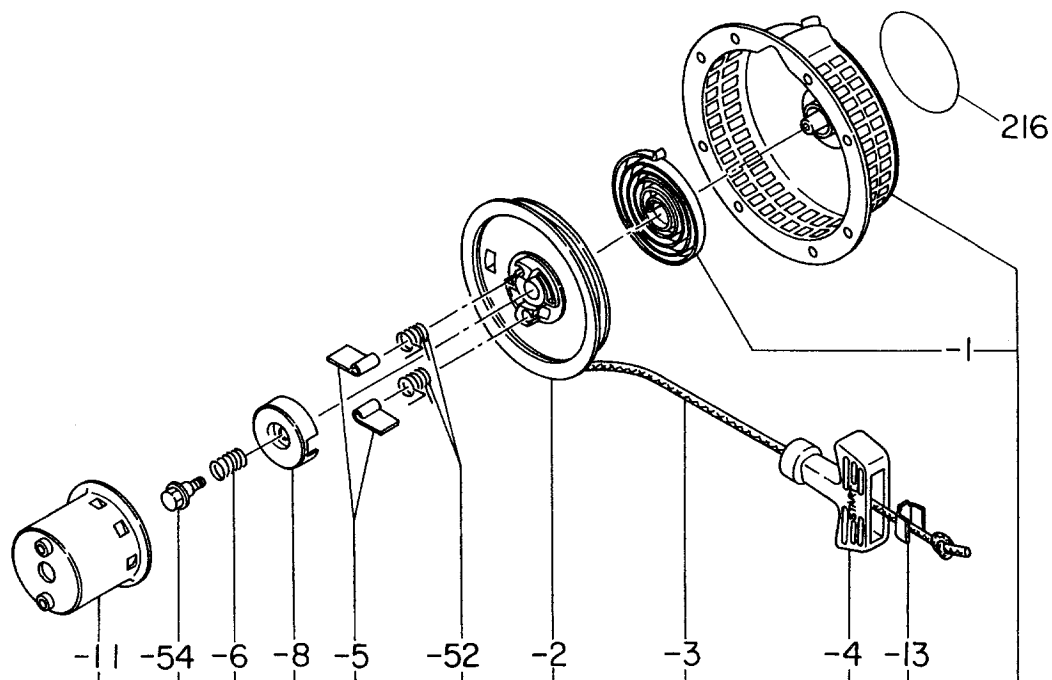
FIG. 500 リコイルスタータ AY
