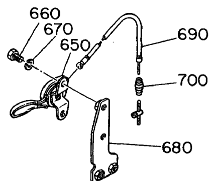
DETAIL(B)TYPE
