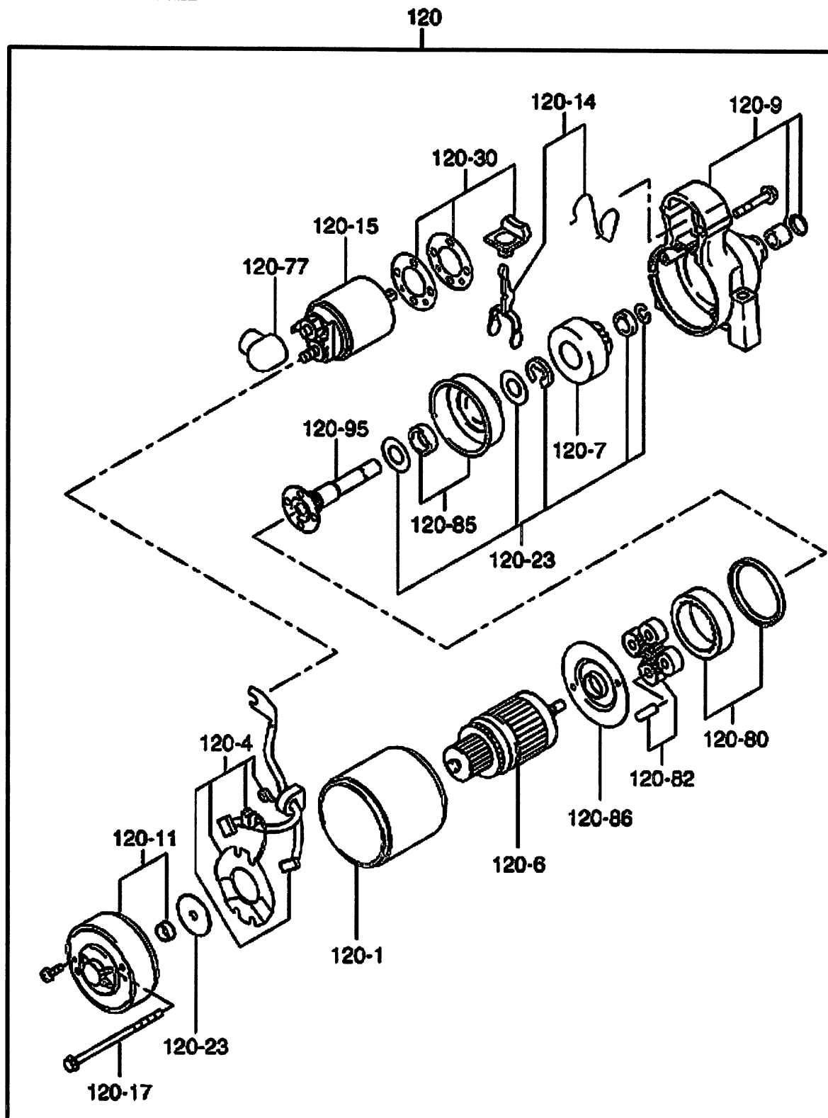
FIG. 731
