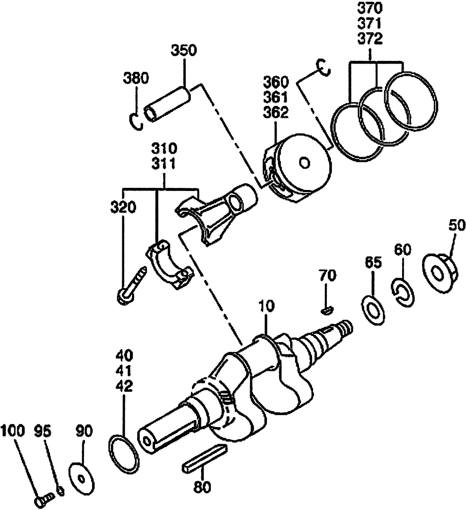
FIG. 200
