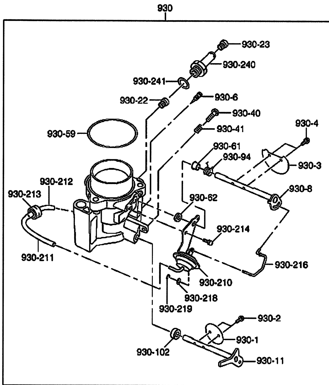
FIG. 650
