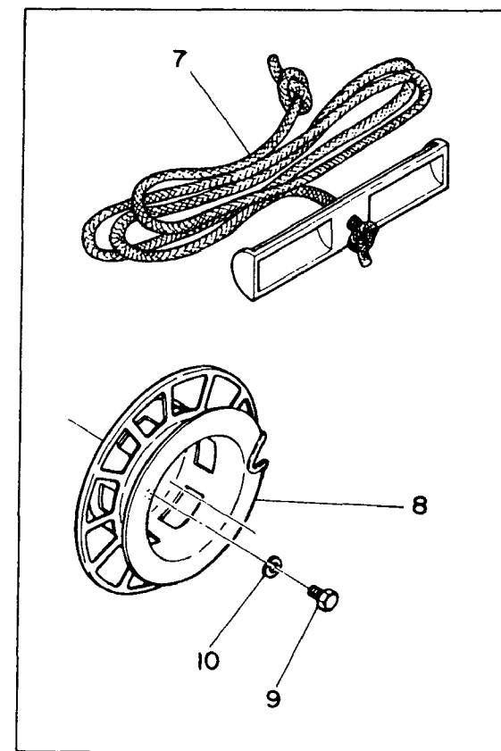
OPTIONAL PARTS
