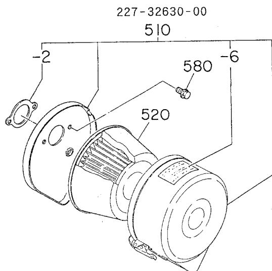
ケロシン用サイクロン形
