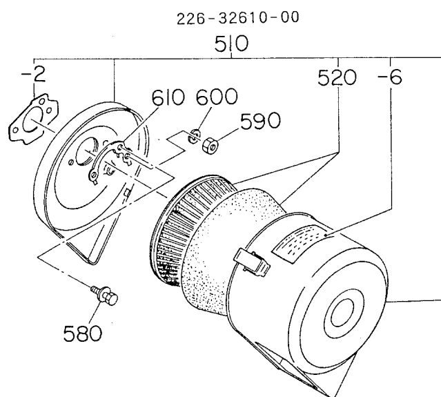
サイクロン形
