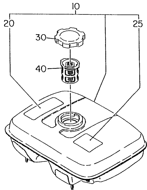
プレート用タンク TANK, for PLATE
