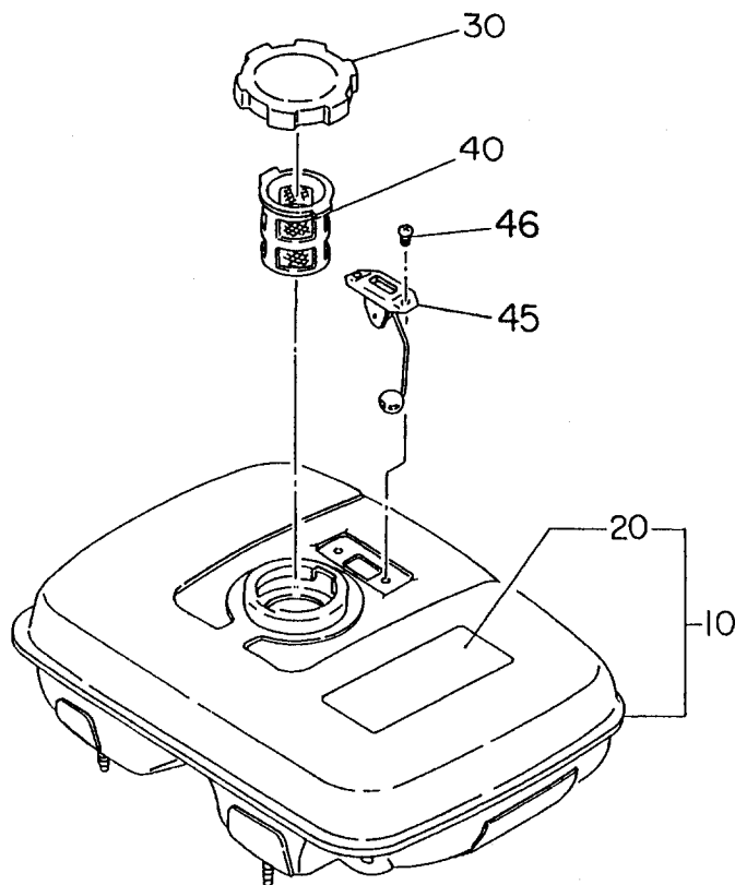
B形用タンク (フロートゲージ式) TANK, for B type (FLOAT GAUGE type)
