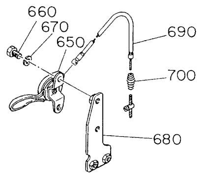
DETAIL(B) TYPE
