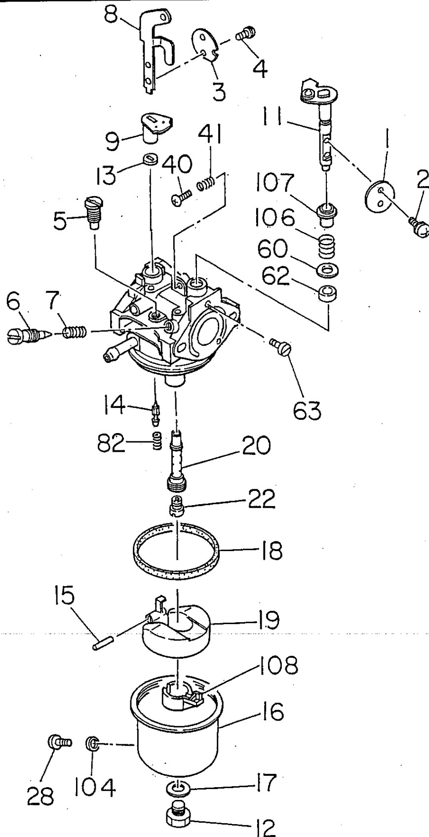
FIG. 6200 キャブレータ AY CARBURETOR AY
