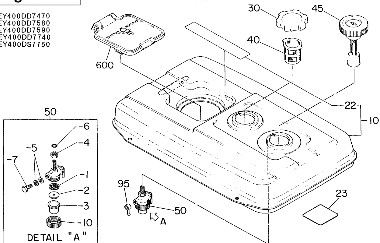
ゲージ付タンク (キャップ式)
