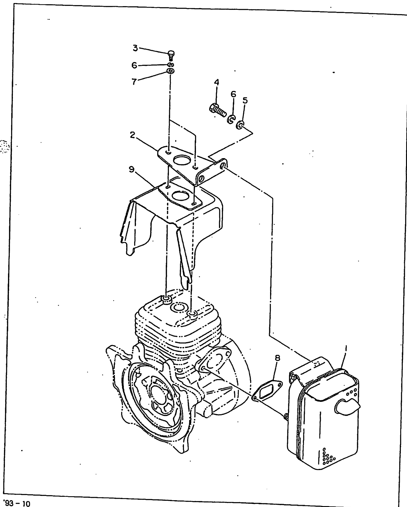
FIG. 3 MUFFLER
