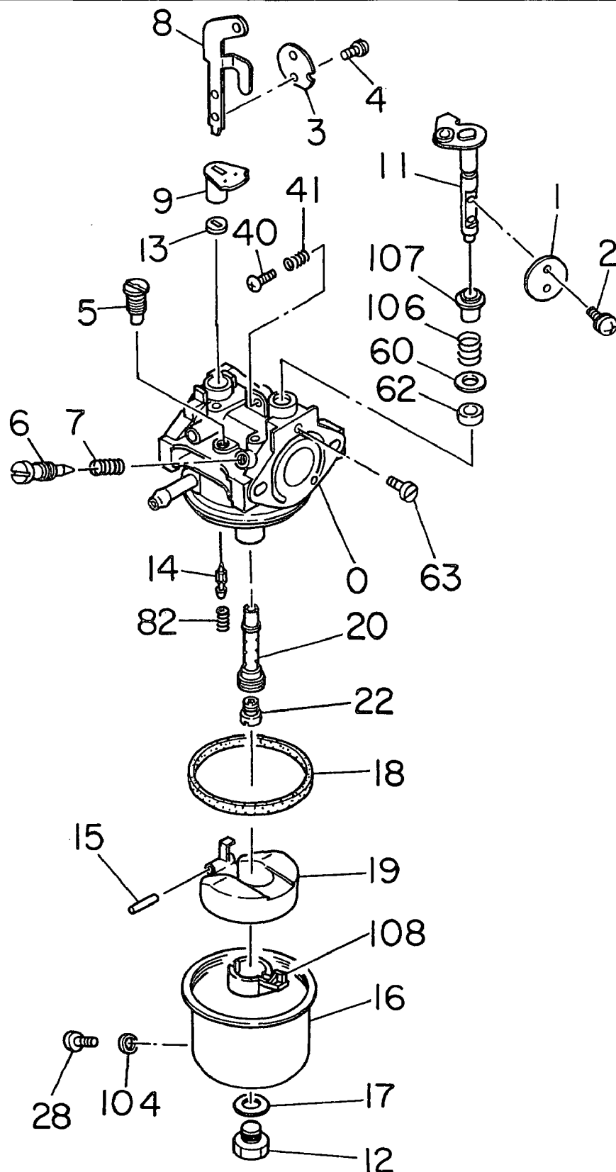
FIG. 6200 キャブレータ AY-2 CARBURETOR
