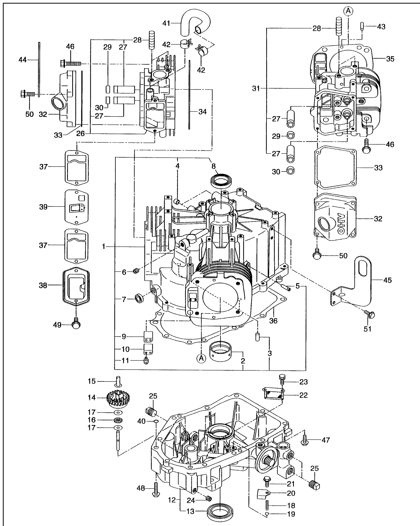
FIG. 1 CRANKCASE GROUP - EH63V / EH65V
