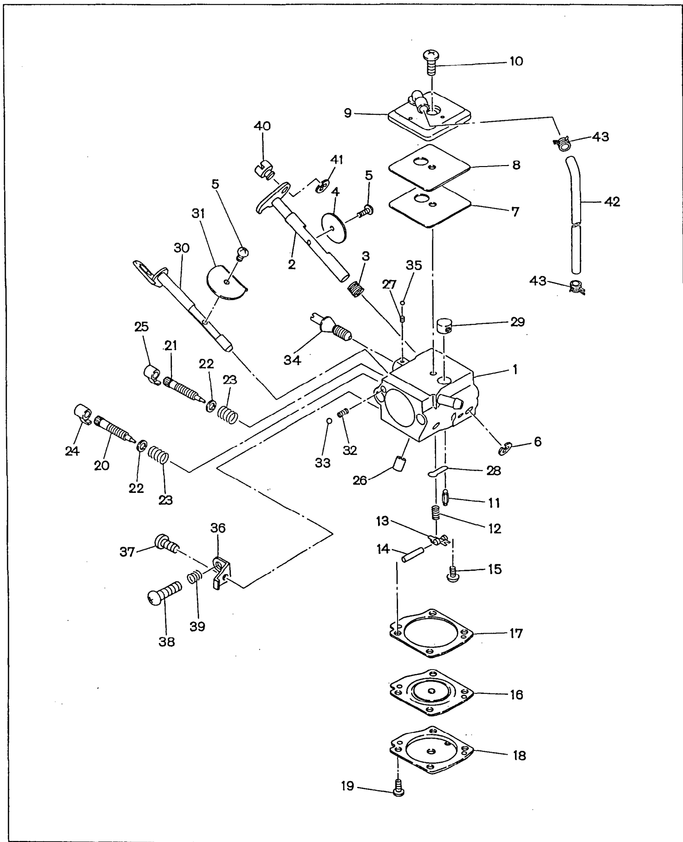
FIG. 5 CARBURETOR
