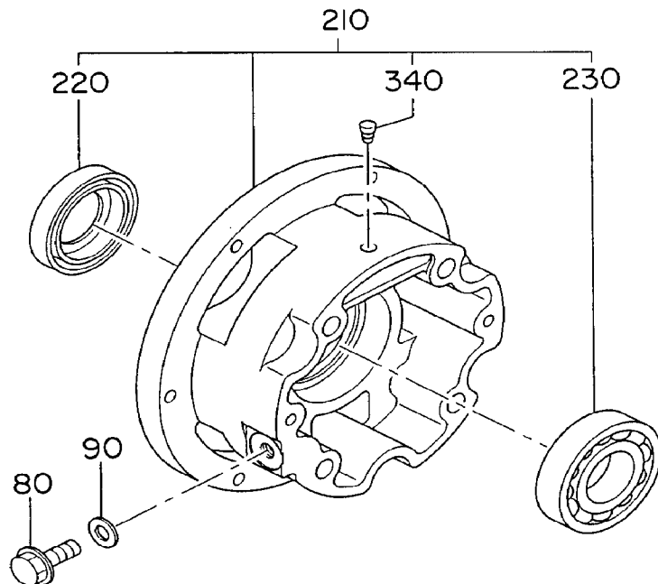
クランクケース カバー CRANKCASE COVER
