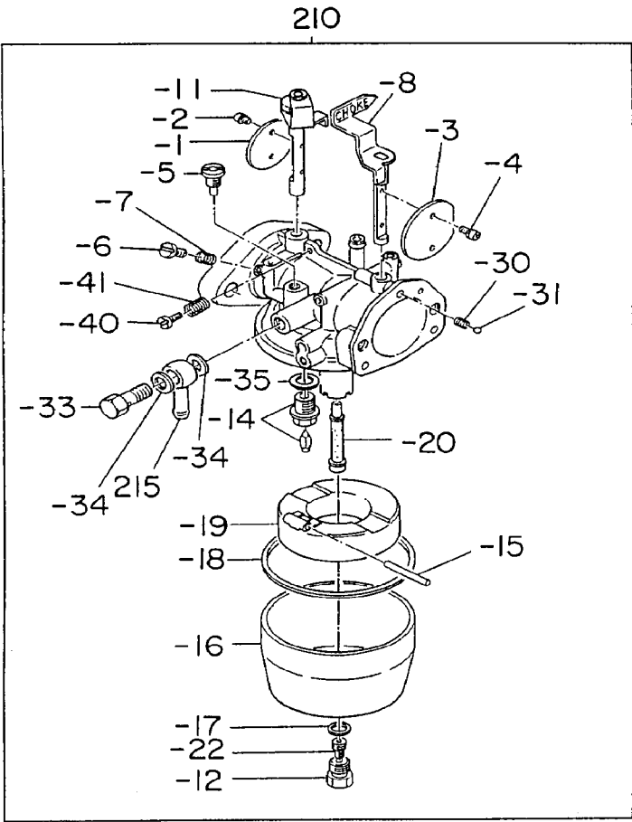
キャブレータ AY CARBURETOR AY
