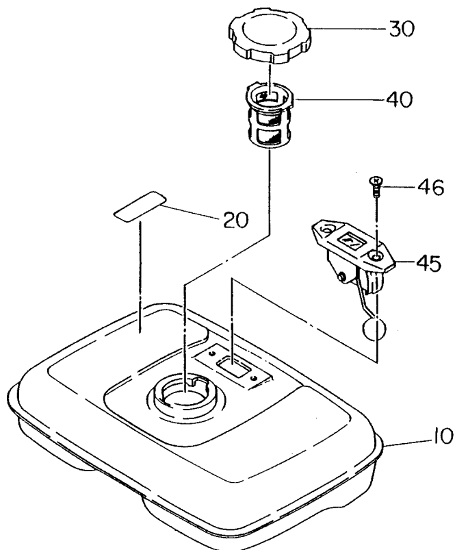
フロート ゲージ付 W/FLOAT GAUGE
