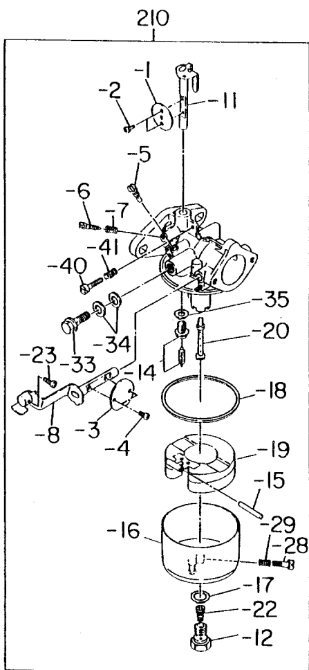
ドレイン付 W/DRAIN
