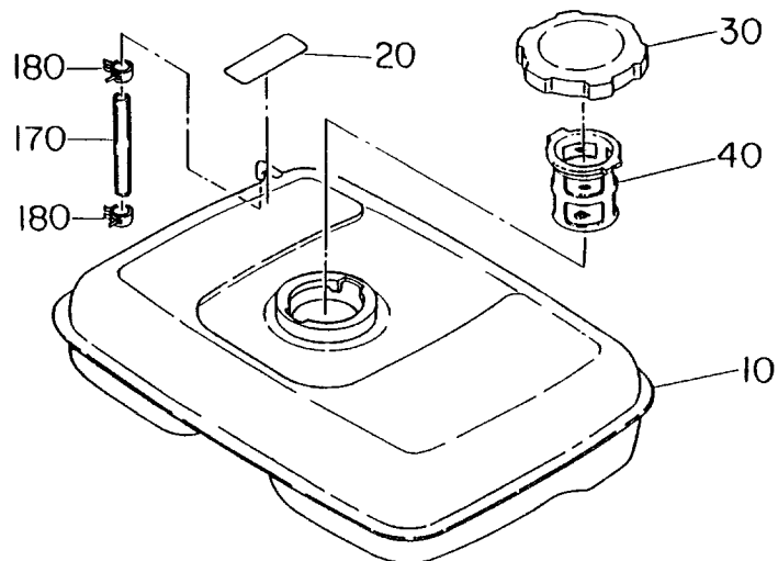
ビニール パイプ ゲージ付 W/VINYL PIPE GAUGE
