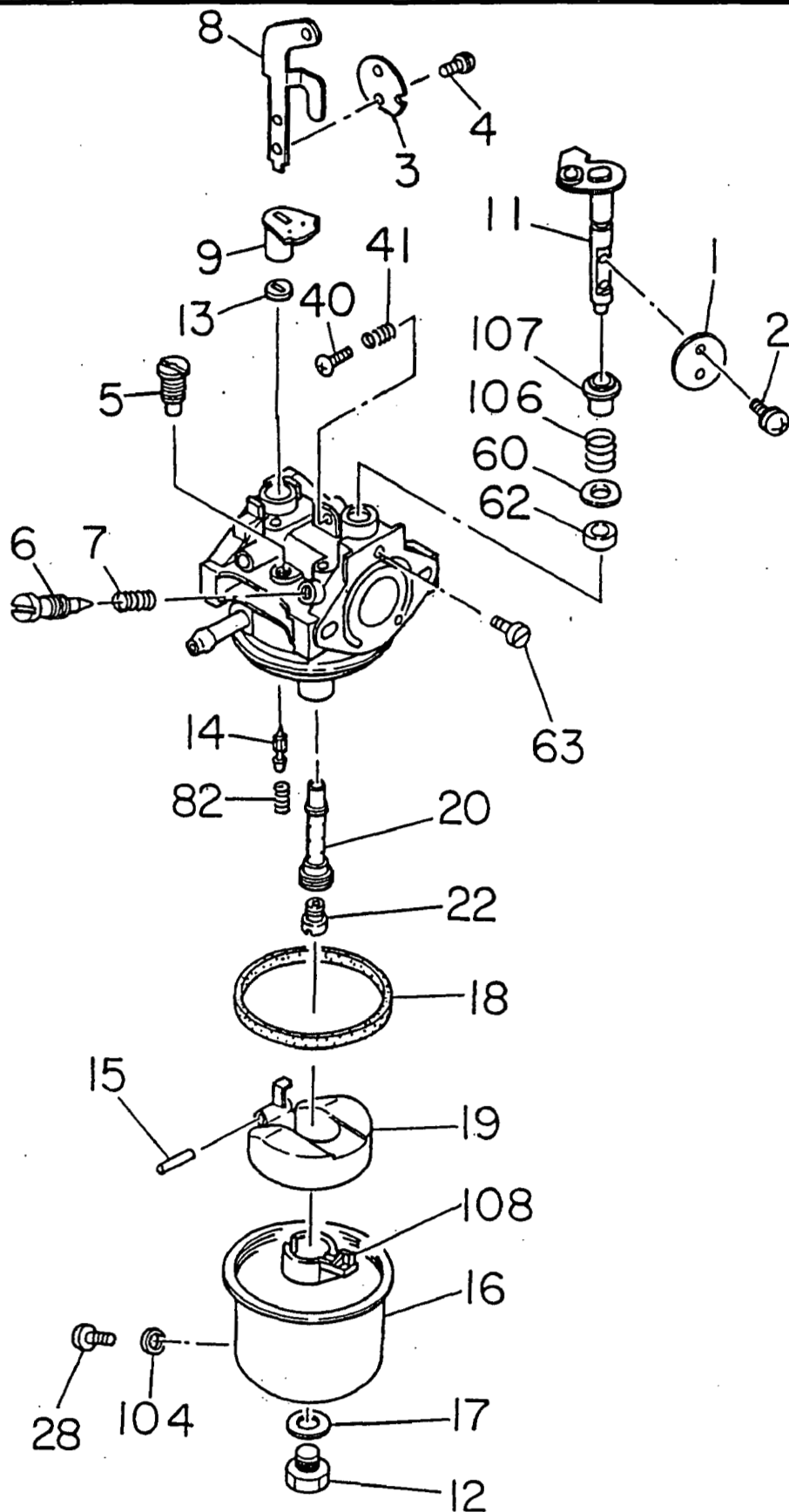
FIG. 6200 キャブレータ AY CARBURETOR AY
