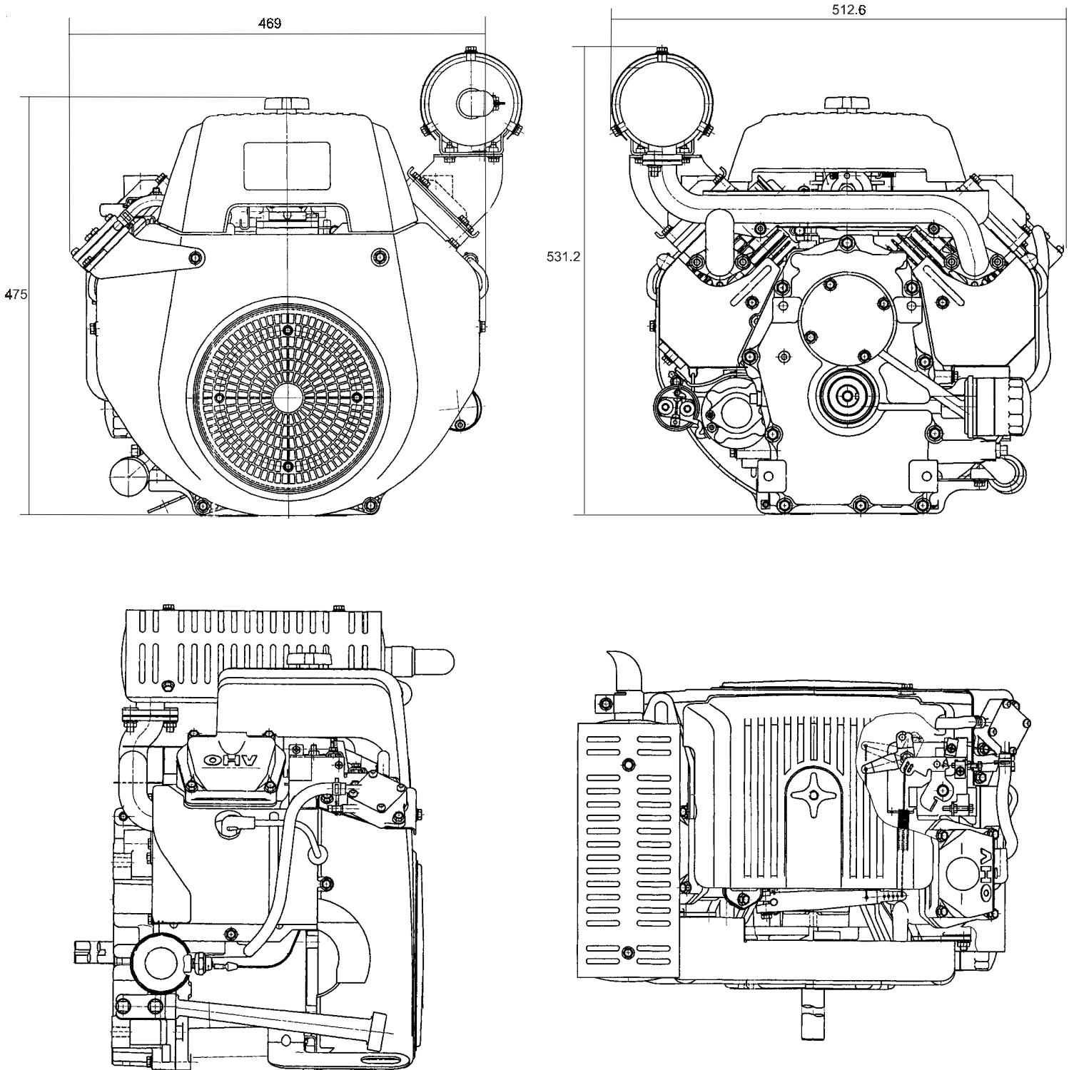
92630014 - Muffler
